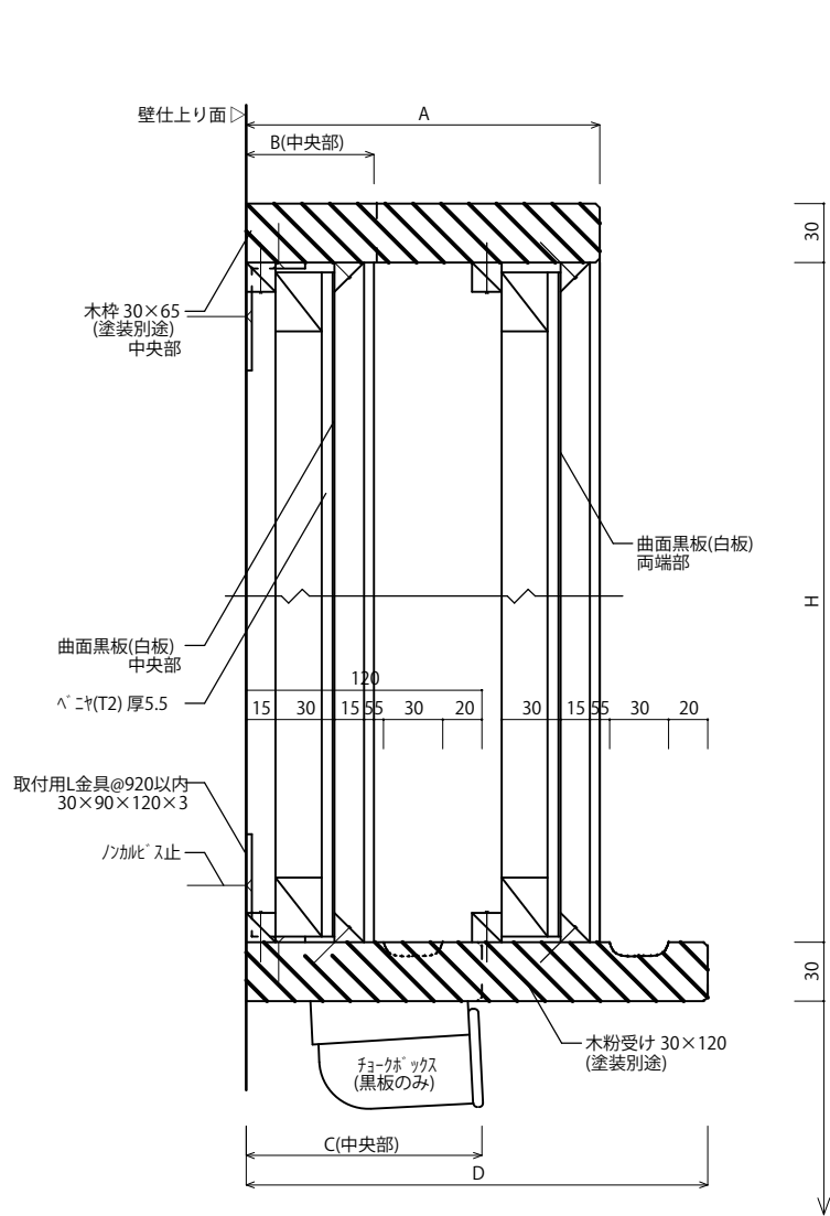
断面図 1/3
