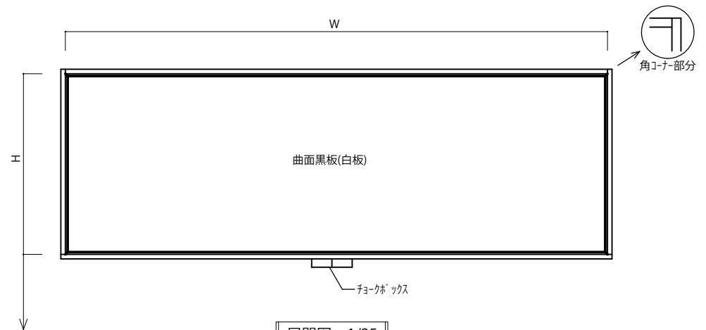
展開図 1/25
