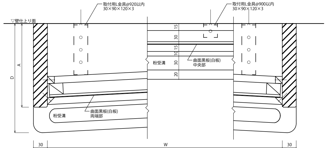
断面図 1/3
