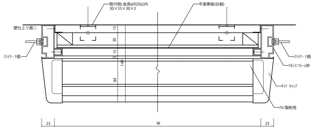
平面図 1/3
