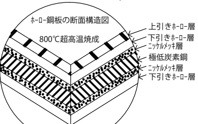
断面図 1/3
