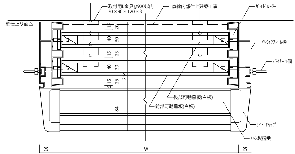
平面図 1/3
