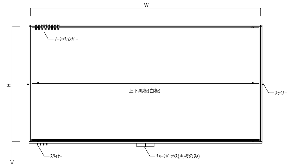
展開図 1/25
